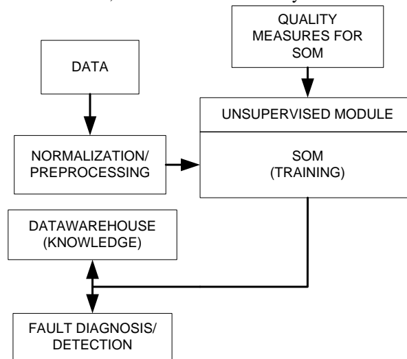
Fig. 6. The component interaction between SOM
